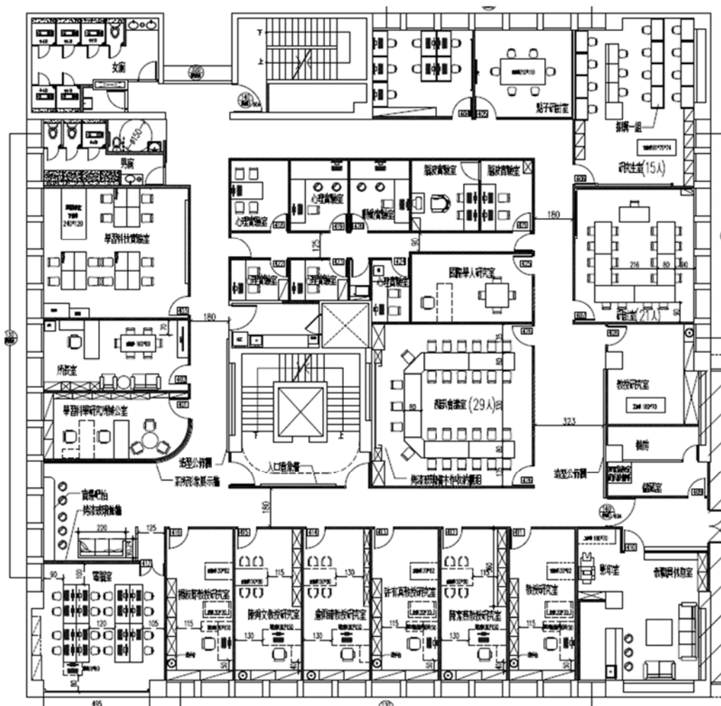
圖 1 學科所於綜二館 4 樓空間平面規劃圖
